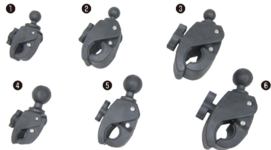
●タフクランプ ①RAP-B-400U パイプクランプ径16～38mm、ボール径25mm ②RAP-B-404U パイプクランプ径25～47mm、ボール径25mm ③RAP-B-401U パイプクランプ径16～57mm、ボール径25mm ④RAP-400U パイプクランプ径16～38mm、ボール径38mm ⑤RAP-404U パイプクランプ径25～47mm、ボール径38mm ⑥RAP-401U パイプクランプ径25～57mm、ボール径38mm
