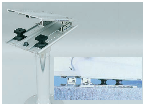
●77000 シートサスペンション ・シートとベディスタル、シートスライド間での使用 ・直接フロアーに付けボートシート間での使用
